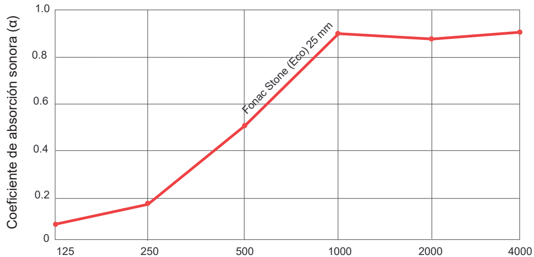
Curvas de atenuación sonora
