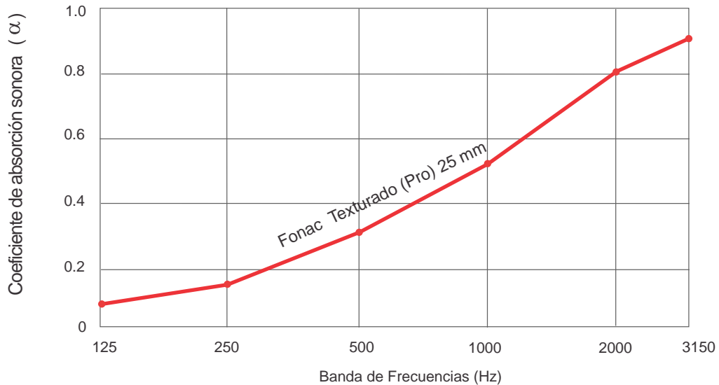
Curvas de atenuación sonora
